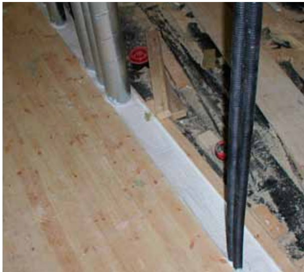
Figur 30 Exempel på genomföring i bjälklag.
