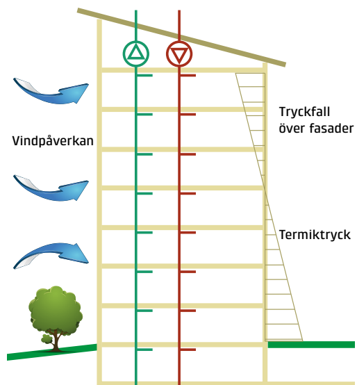
Figur 33 Exempel på tryckskillnader som kan uppstå i ett flervåningshus.
